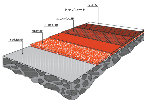
ウレタン舗装詳細図
