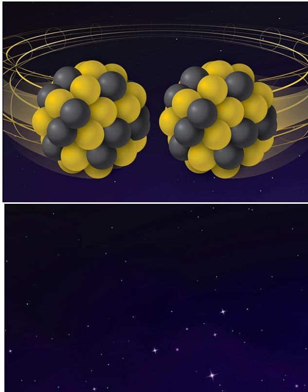
RHIC: 相対論的重イオン衝突型加速器
