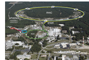
RHIC@BNL
