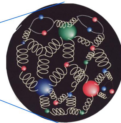
クォークと グルーオン (TeV)
