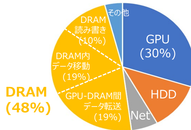
AI時代のGPUサーバの消費電力内訳
