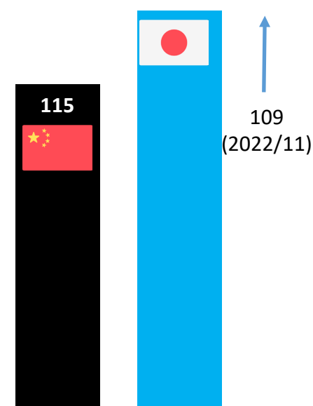
Graph500 (単位：TTEPS)
