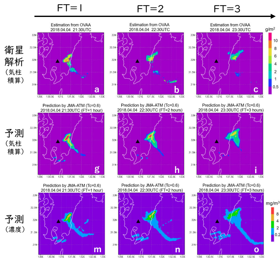
ひまわり8号観測データから作成したJMA-ATMの初期値を用いて火山灰雲の濃度を予測した例（2018年4月4日新燃岳噴火の事例）
