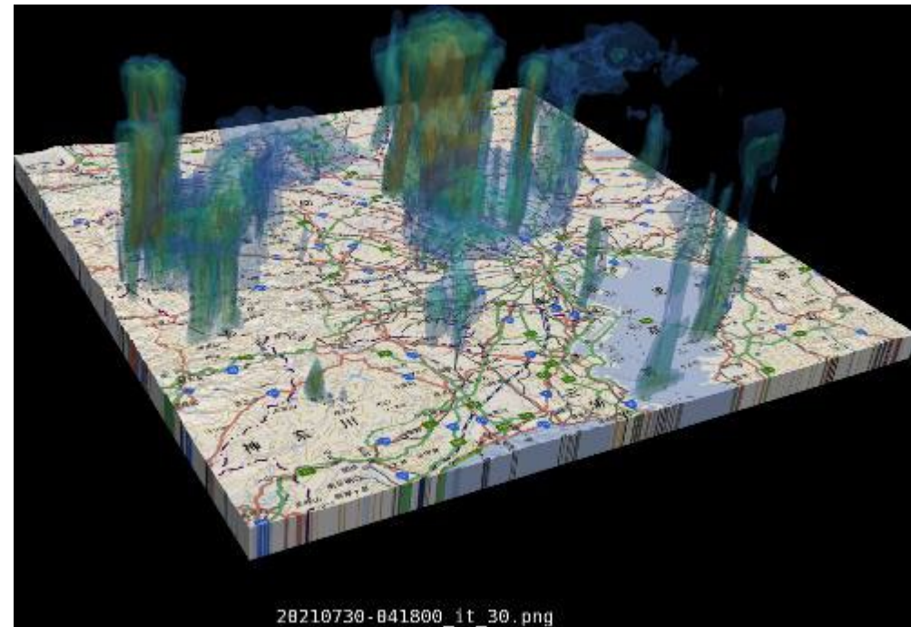
図：2021年7月30日13時18分00秒（日本時間）を初期時刻とする13時33分00秒（15分先）の3次元的な降水分布の予測。色は雨の強さを示す。見やすくするために鉛直方向は3倍に引き延ばしている。国土地理院の地図データを使用した。
