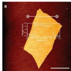
GOナノシートのAFM画像 (スケールバー: 2µm)
