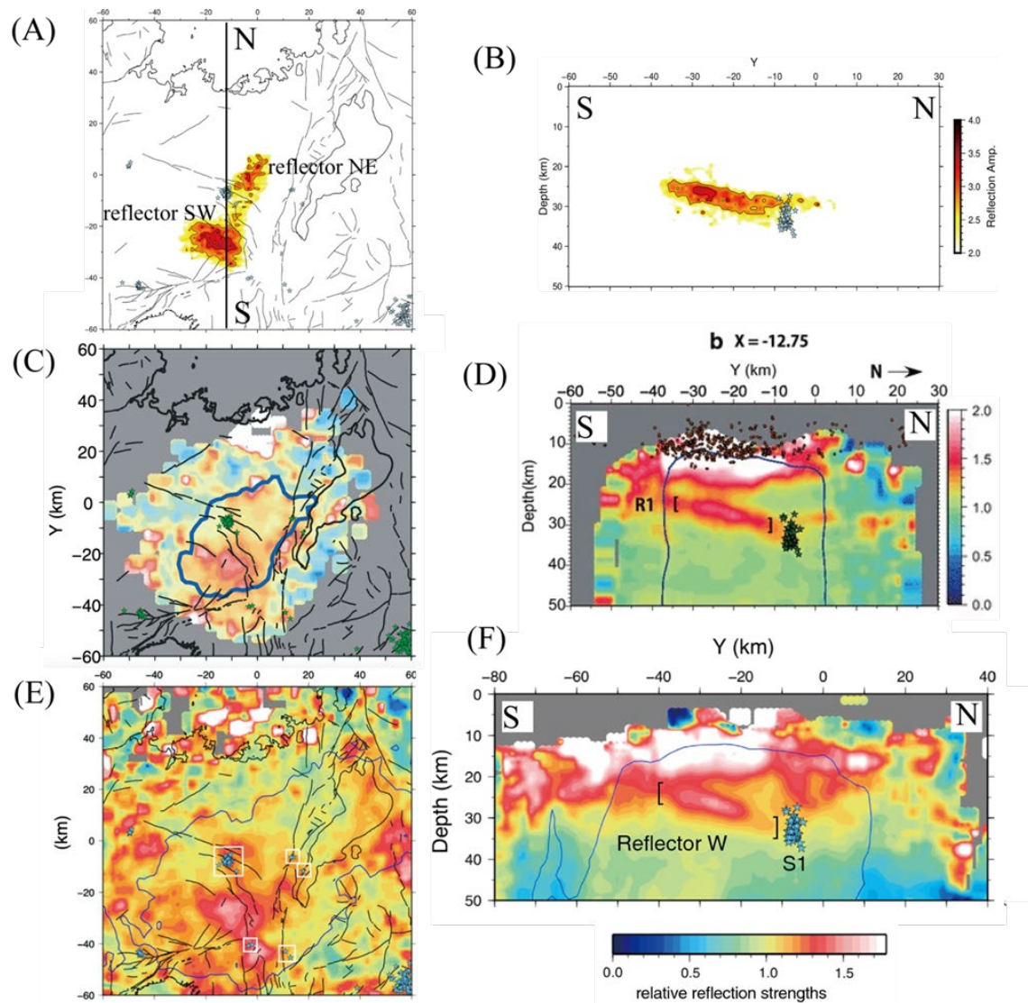
図 8. 有馬高槻断層帯の北方の下部地殻内の S 波の reflector。(A) は深層学習を活用して推定された S 波 reflector の上面、(B) は (A) の測線に沿う南北断面における反射強度の断面図 (加藤, 2022)。一番外側のコンターが reflector とする反射振幅の閾値 (median- \sigma ) に対応している。(C) と (D) は Aoki et al. (2016)、(E) と (F) は Katoh et al. (2018) の結果。(B)、(D)、(F) は (A) 上の測線の南北断面図。各図の星印は気象庁一元化震源における深部低周波地震。(D) の赤い丸印は測線から幅 5 km 以内で Aoki et al. (2018) が解析に使用した地震、青い線はグリッドに含まれるデータ数が 50000 個の等値線。(E) および (F) の青い線はグリッドに含まれるデータ数が 10000 個の等値線。黒線は活断層 (京都大学防災研究所 [課題番号: DPRI03]、中田・今泉, 2002)。
