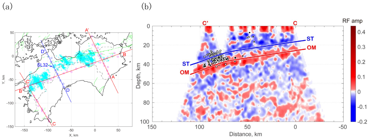
図6. (a) 測線図。(b) 測線CC'におけるレイリー関数イメージ。レイリー関数の正の振幅を赤で、負の振幅を青で示す。STとOMを付した線は、それぞれフィリピン海スラブの上面とスラブ内の海洋モホ面と解釈される。白丸は深部低周波時地震、黒丸は通常地震を示す（京都大学防災研究所 [課題番号：DPRI02]）。
