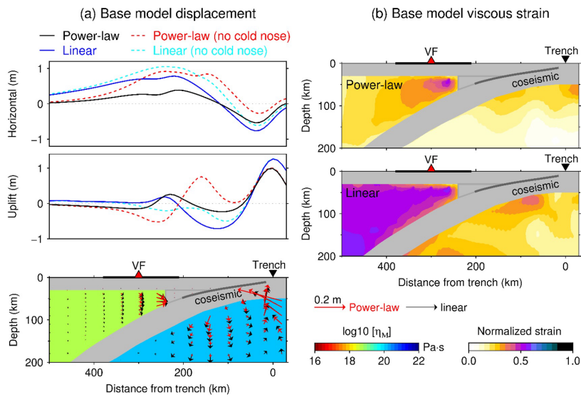
図 13. 非線形レオロジーを使用した余効変動モデル (Dhar et al., 2023)。a) 線形、べき乗レオロジーによる地表変動 (実線はコールドノーズあり、点線はコールドノーズなし)。べき乗レオロジーの方が、震源に近い部分でのみ変形小さい (ただし、両者の定常粘性率はほぼ同じ値を採用している)。b) レオロジーによる粘性歪み分布の違い: べき乗 (上)、線形 (下)。べき乗レオロジーの方が、震源に近い部分で粘性の低下により粘性歪が発生するが、線形モデルではモデル領域全体で変形している。これが a) での全体の変形量の幅を決めている (東北大学理学研究科 [課題番号: THK_07])。
