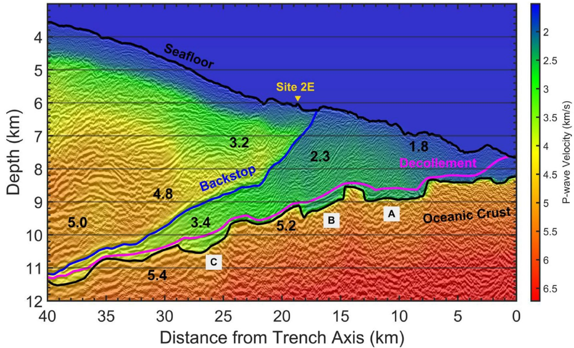
図2. 東北沖の日本海溝を横切る反射法探査測線 D13 の地殻構造と P 波速度構造モデル。図中の数字は P 波速度、A、B、C はグラバーン構造（東京大学大気海洋研究所[課題番号：AORI01]）。
