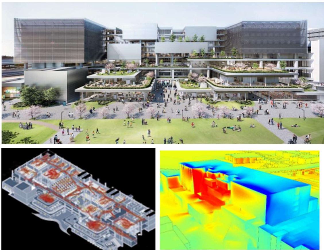
(図3) 学部・研究科の移転にあわせて新設する施設において、人流や温湿度等の各センシングにより、省エネルギーの最適運用と交流の誘発や環境意識向上等に向けた可視化を実現し、省エネルギーとイノベーションを両立する次世代型エコキャンパス計画を構想（立命館大学・大阪いばらきキャンパス）
