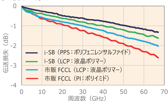
i-SB法 ® で作製した基板と市販基板の伝送損失
