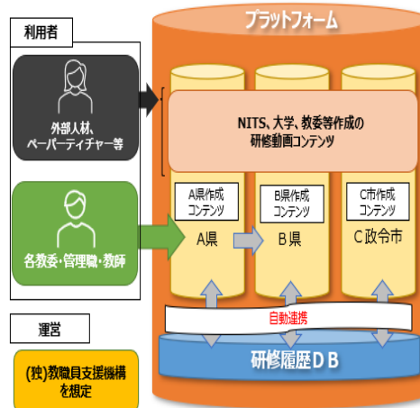
<研修受講履歴記録システム構築イメージ>
