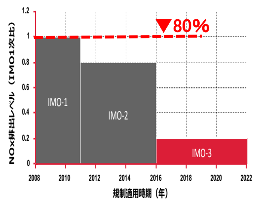
NOx国際規制の強化(日本提案)
