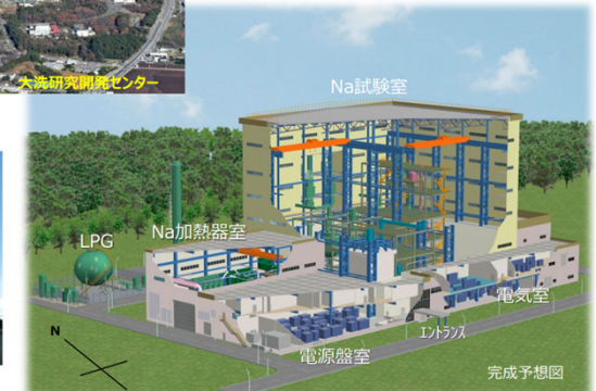
完成予想図
