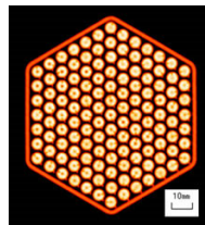
燃料集合体 X線CT画像
