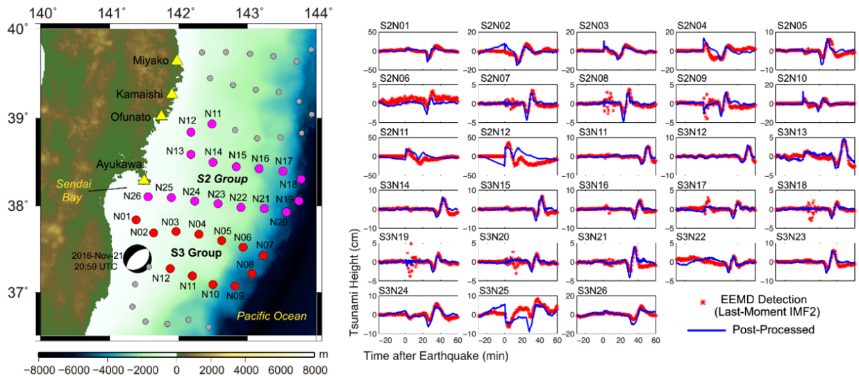
図 13. 2016年福島県沖の地震 (M7.4) に対するデータ同化による津波波動場の現況把握ならびにそれに基づく津波即時予測の実データへの適用。(弘前大学工学研究科 [課題番号: HRS_02])
