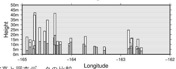
沿岸での計算最大波高と調査データの比較
