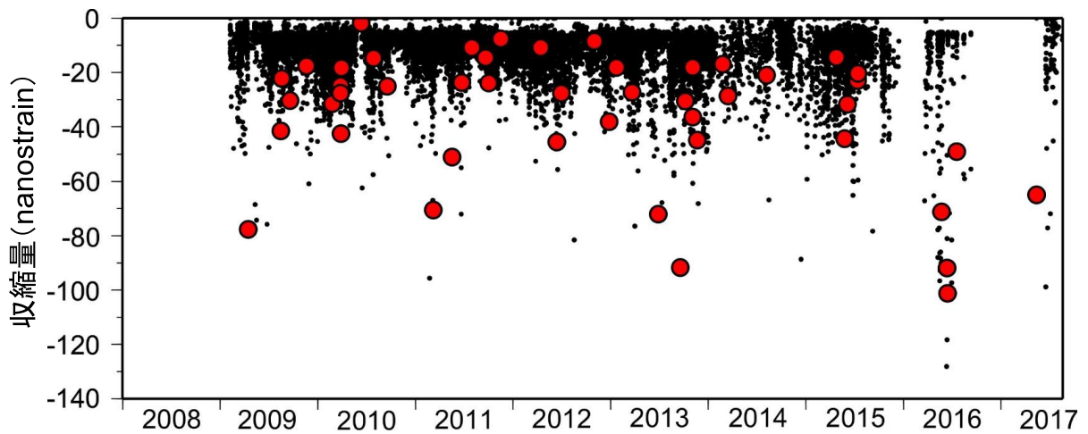
図 11. 桜島火山 有村観測坑道伸縮計 T 成分時系列データと火砕流の発生との比較。火砕流をとともう噴火は収縮量が大きい。すなわち噴出物が多い噴火の際に火砕流が発生しやすい。（京都大学防災研究所 [課題番号：DPRI11]）
