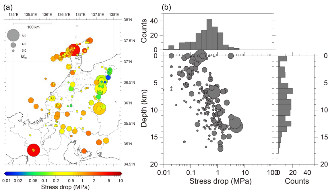
図 1. 北陸地方で発生した地震に対して、スペクトルインバージョンで得られた震源項に \omega^{-2} スペクトルモデルを当てはめ、コーナー周波数と円形クラック半径の関係 (Brune, 1970,
