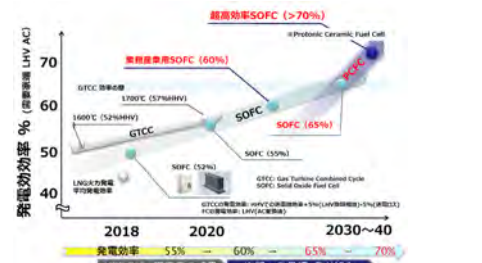
燃料電池効率向上に向けたNEDOの取り組み
