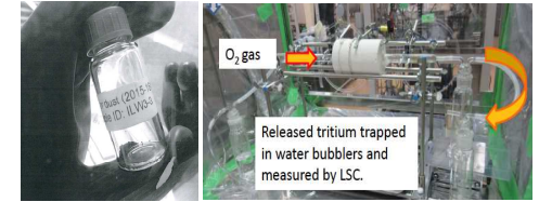
大型トカマク装置JET(英国)のタイルとダストの分析
