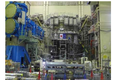
組立が完了したJT-60SA
