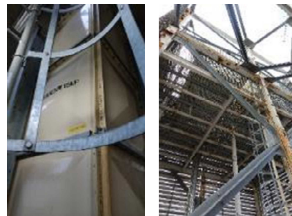
高架水槽の状態 (高架水槽壁内)
