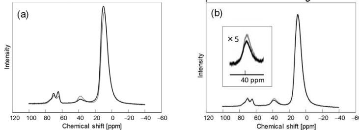
(a) I-NaOH-6.3-85 (黒色実線)とI-NH3-8.6-90 (灰色実線)と、(b) MO吸着前のI-NH3-8.6-90 (灰色実線)と吸着後(黒色実線)の 27 Al固体NMRスペクトル。挿入図に5配位付近を拡大して示す。
