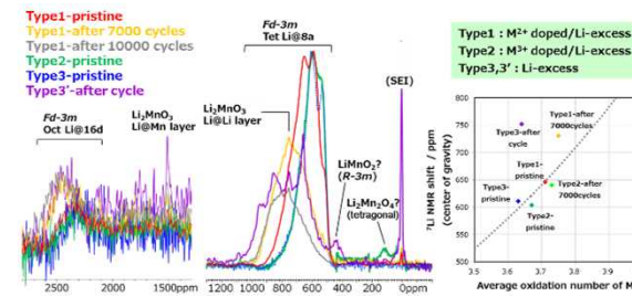
スピネルMn系正極材の 7 Li MATPASS 解析結果
