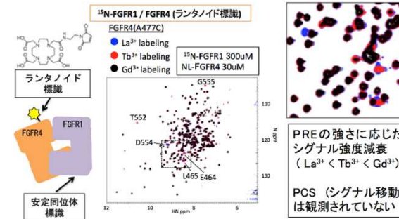
Tb 3+ によるPREの観測
