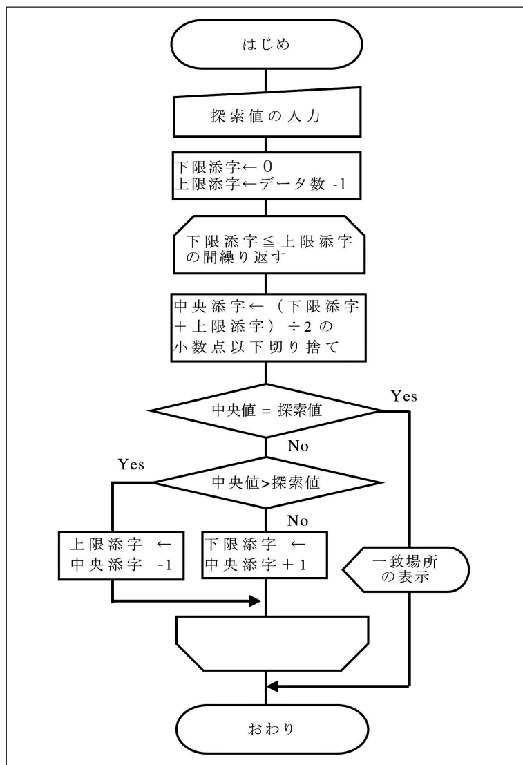
図表5 二分探索
