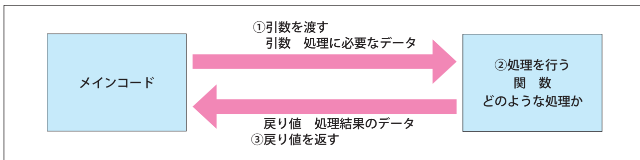
図表 6 プログラムにおける関数
