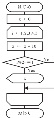
図表 14 流れ図
