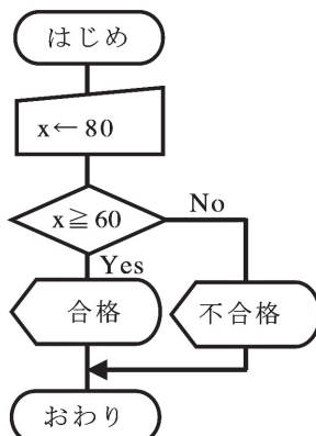
図表8 流れ図
