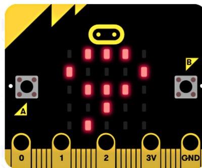
図表 8 反復
