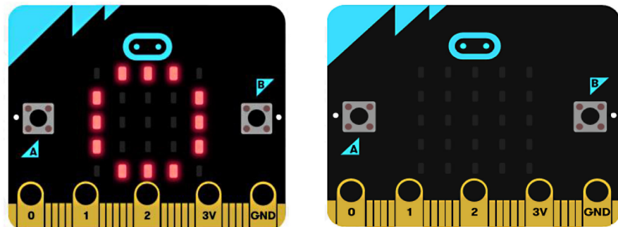
図表 6 順次
