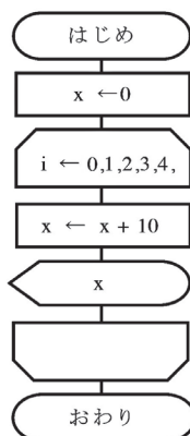
図表 11 流れ図
