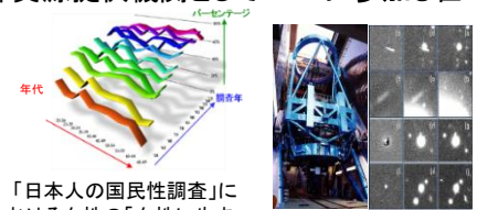
すばる望遠鏡における可視光突発天体の選別
