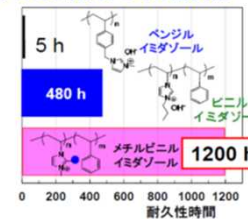
アルカリ水、80°Cでの耐久性
