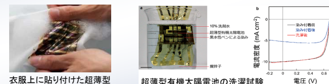
衣服上に貼り付けた超薄型有機太陽電池の洗濯写真
