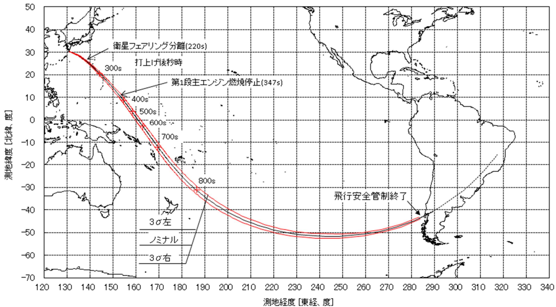
図6 ロケットの落下予測点 (注) 軌跡と3σ分散範囲
