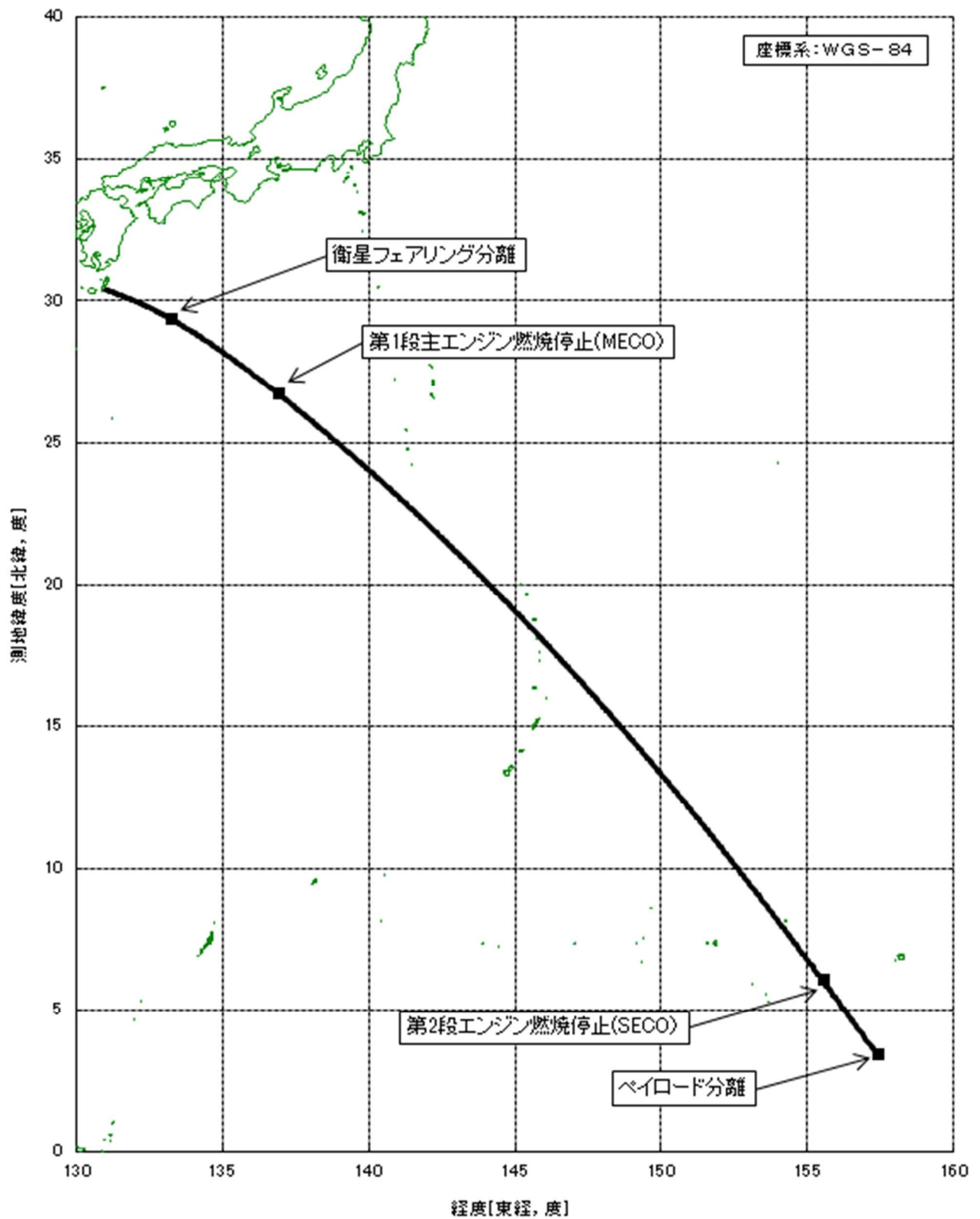
図1 H-IIBロケット7号機の飛行経路概要(機体現在位置)
