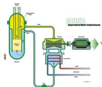
超臨界圧水冷却炉 (SCWR)
