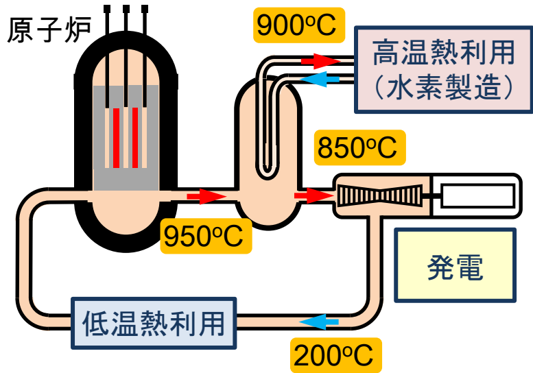
熱電併給用高温ガス炉システム
