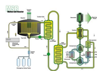
溶融塩炉 (MSR)
