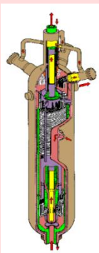
中間熱交換器
