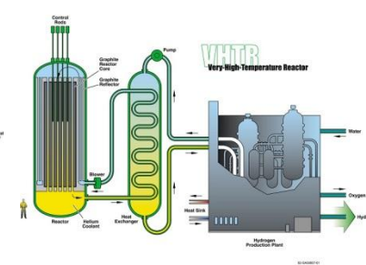
超高温ガス炉 (VHTR)
