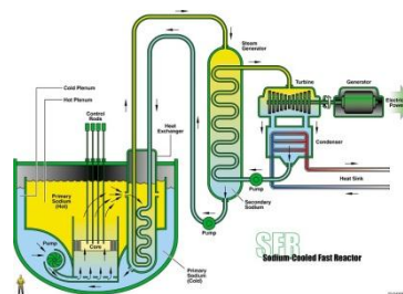
ナトリウム冷却高速炉 (SFR)
