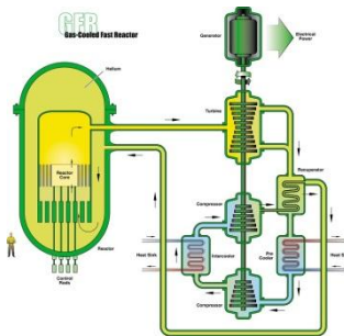
ガス冷却高速炉 (GFR)
