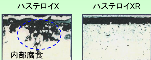
1000°C 10000hr腐食試験後断面写真
