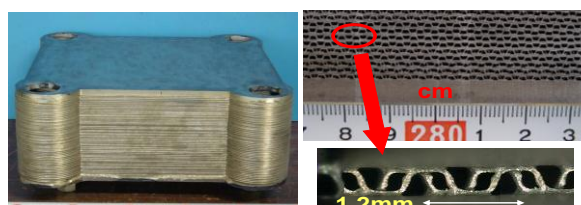
熱交換器本体
