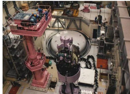
HTTRの外観および内部
