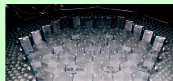
炉内黒鉛構造物
