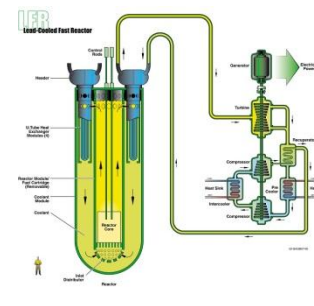
鉛冷却高速炉 (LFR)
