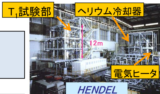
HENDELの外観
