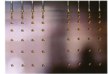
燃料核の振動滴下-外部ゲル化法
