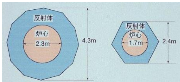
HTTR(左)とVHTRC(右)の炉心断面図
