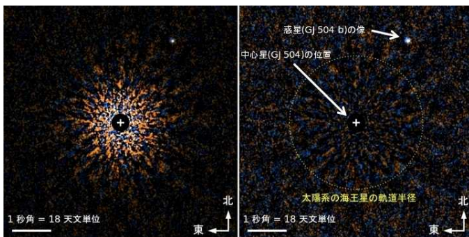
すばる望遠鏡が捉えた、太陽型恒星 GJ 504 のまわりの低質量惑星
