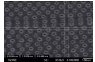
微小ビット列のSEM像:ビットサイズ 35\text{nm}\times 50\text{nm} 、 ビットピッチ 100\text{nm} 、 トラックピッチ 50\text{nm}
