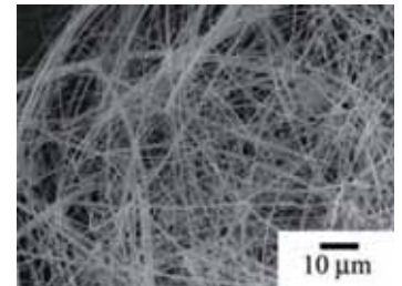
本製法で作成した炭化ケイ素ナノファイバの 電子顕微鏡写真
