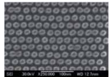
微小ビット列のSEM像:ドット径 13\text{nm} 、 ビットピッチ 25\text{nm} 、 トラックピッチ 25\text{nm}
