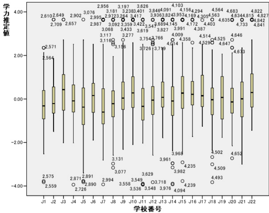
図 5-10 各学校における学力推定値（ \theta ）の箱ひげ図（中学校）
