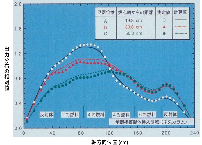
図1 実験値と計算値の比較の例(④出力分布(軸方向))
