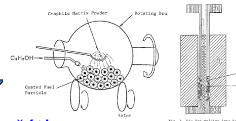
コンパクト成形技術
