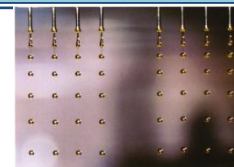
燃料核の振動滴下-外部ゲル化法
