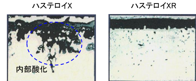
1000°C 10000hr腐食試験後断面写真
