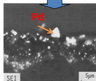
PdによるSiC層の腐食
