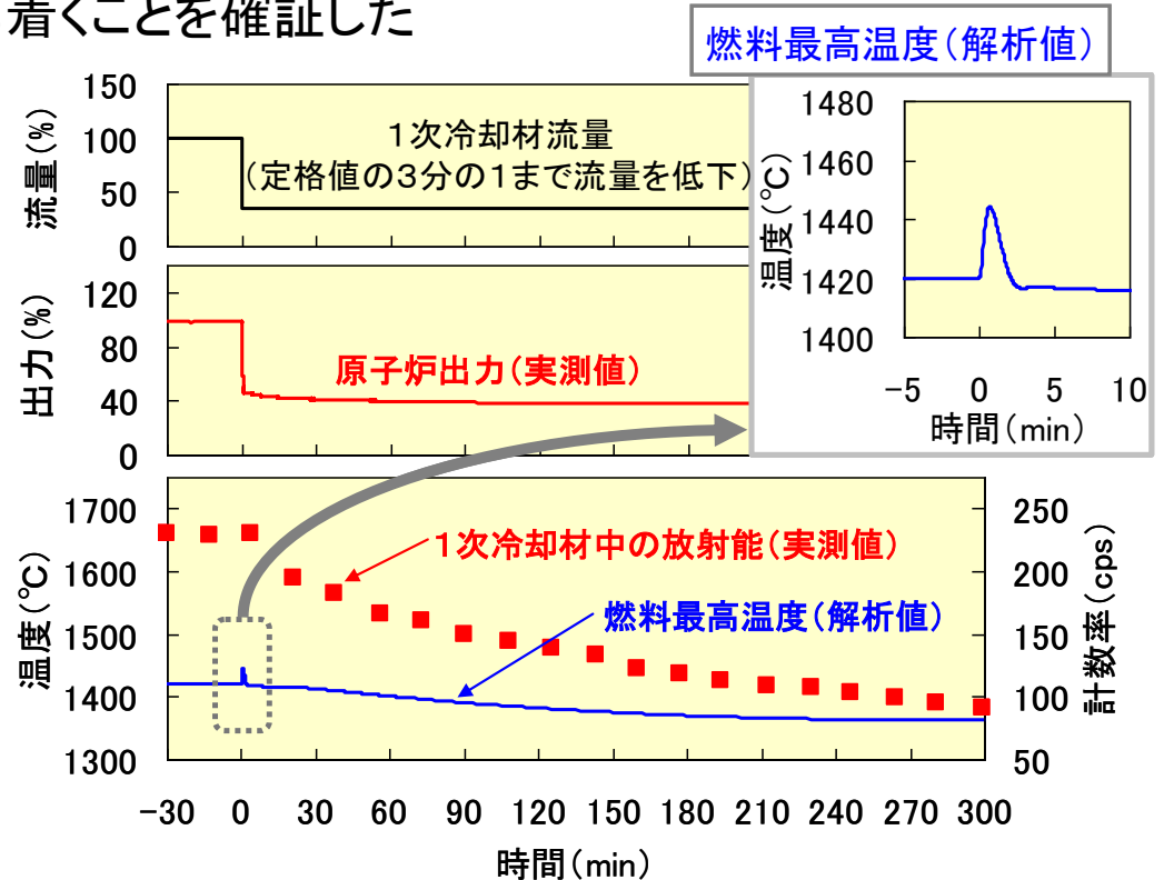
ガス循環機2台停止の結果(原子炉出力100%)
