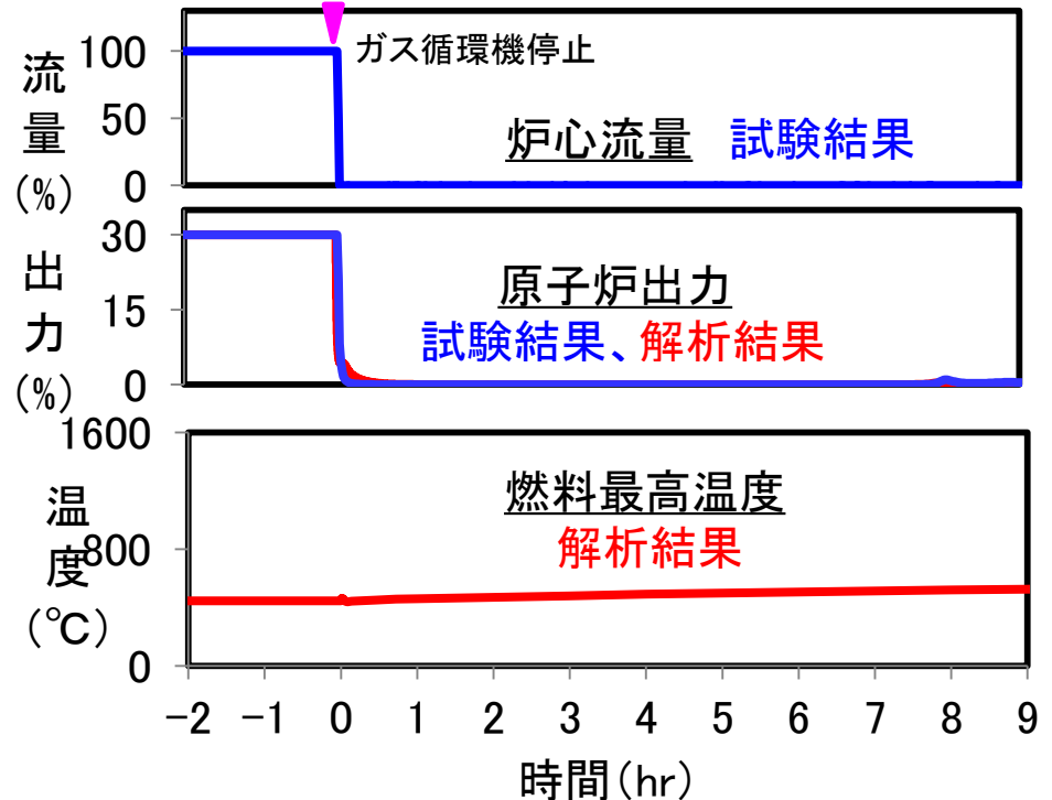
試験及び解析(原子炉出力30%)
