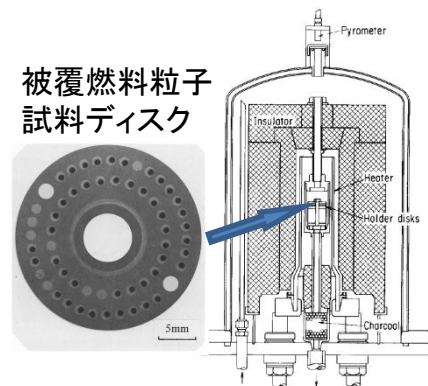
照射後加熱試験装置 (加熱温度: ~2400°C)
