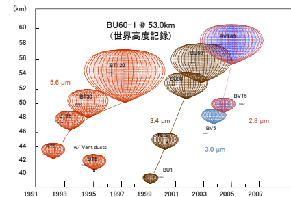
薄膜高高度気球開発の経緯
